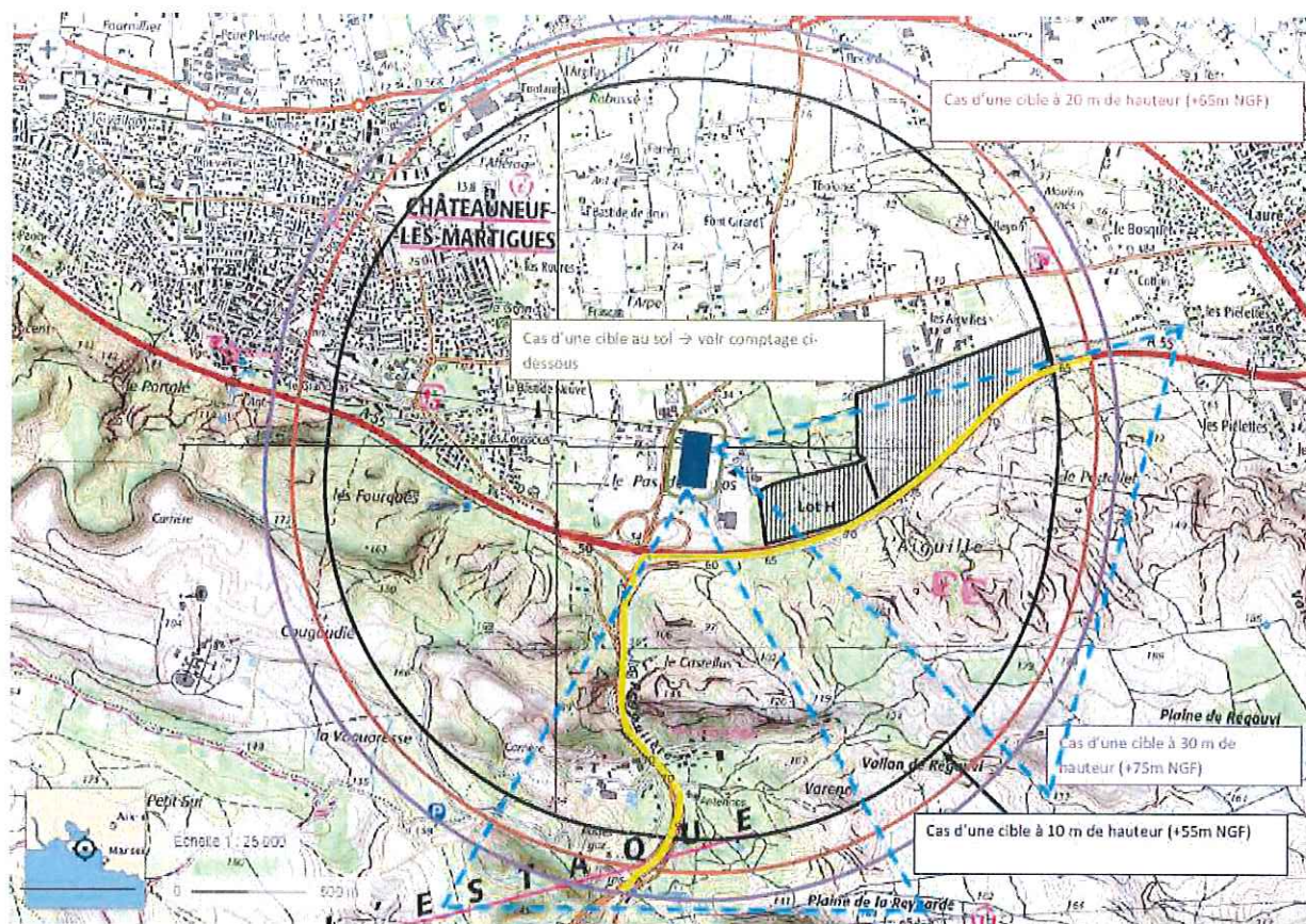
Figure 5 : Représentation des effets toxiques (distance atteintes pour le seuil des effets irréversibles) – Avec représentation des différentes cibles en hauteur
