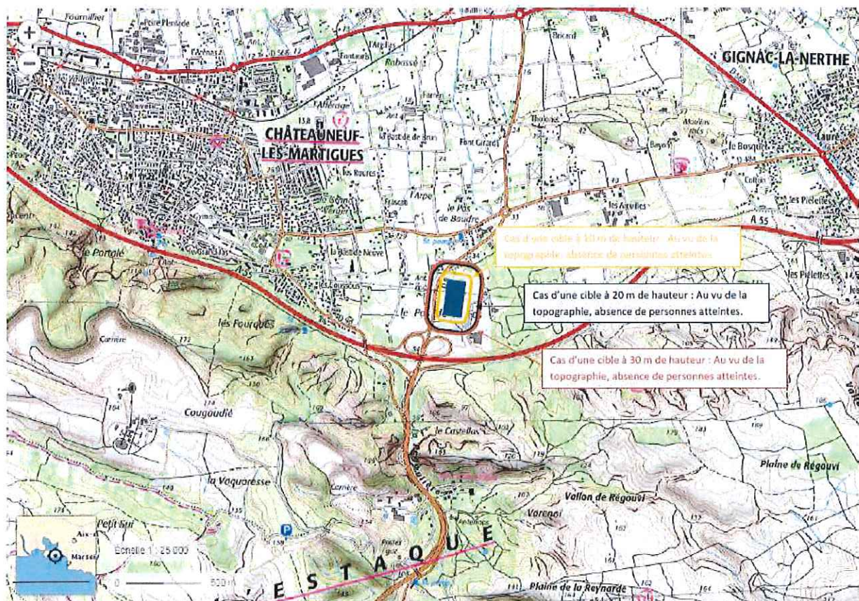
Figure 4 : Représentation des effets toxiques (distance atteintes pour le seuil des effets létaux) – Avec représentation des différentes cibles en hauteur.
